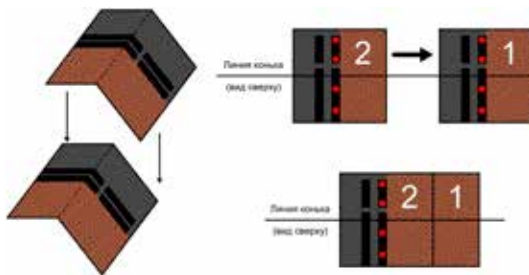
Рис. 26 Устройство рёбер скатов и коньков.
