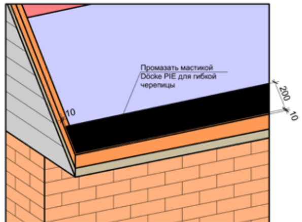
Рис. 16 Герметизация карнизного свеса под укладку ламинированной черепицы Döcke PIE PREMIUM коллекции «Dragon».
