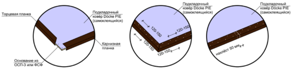
Рис. 8 Крепление металлических карнизных и торцевых планок.
