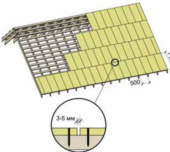
Рис. 5 Укладка сплошного основания из плит ОСП-3 или фанеры ФСФ по обрешётке.
