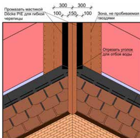
Рис. 20 Выполнение открытой ендовы.
