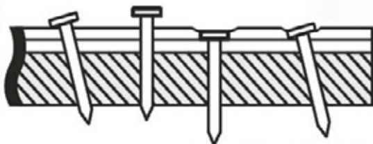
Рис. 3 Пример неправильной забивки гвоздей при монтаже продукции.
