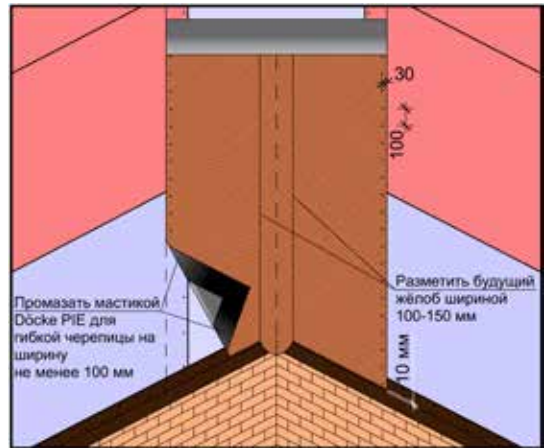
Рис. 9 Монтаж ендового ковра.
