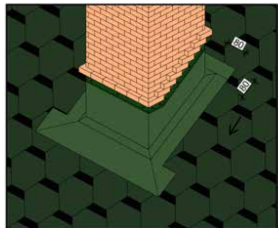
Рис. 22 Примыкание кровли к трубе дымохода.
