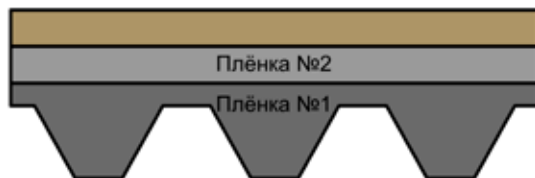
Рис. 13 Тыльная сторона гонта гибкой черепицы Döcke PIE.
