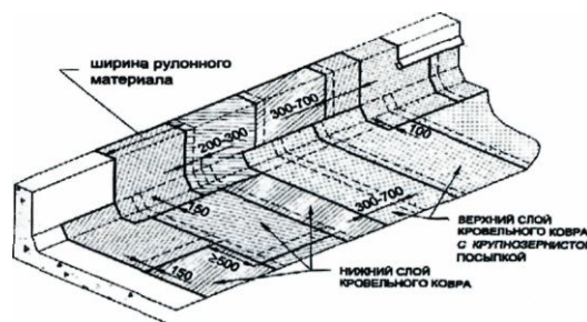
б) схема раскладки полотнищ;
