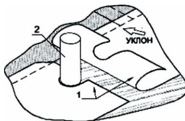
1 - полотнища рулонного материала; 2 - труба.
