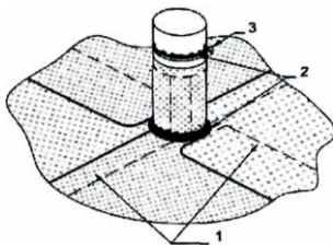
1 - полотнища основного ковра; 2 - герметик; 3 - хомут.
