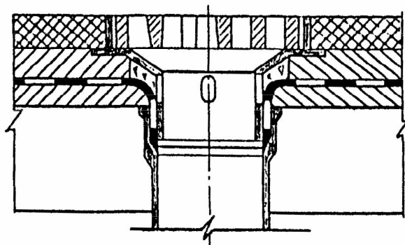
Рисунок 38. Сопряжение гидроизоляции с водоотводной трубкой
