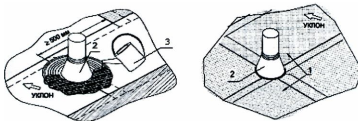
1 - полотнища второго слоя основного ковра «Рубитэкс К-5,0»; 2 - труба; 3 - битумно-полимерная мастика.
