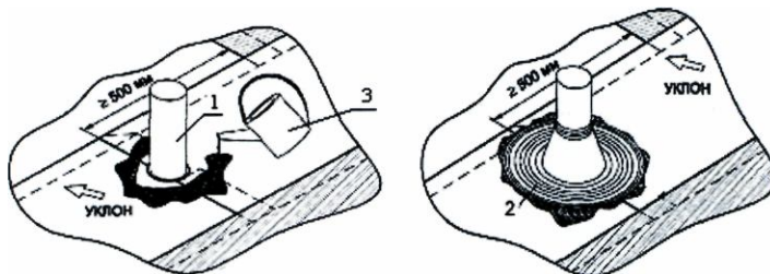
1 - труба; 2 - юбка фасонного элемента; 3 - битумно-полимерная мастика.
