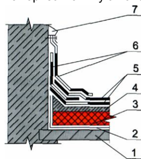
а) схема примыкания;
