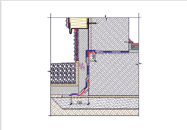
Внутренний угол
