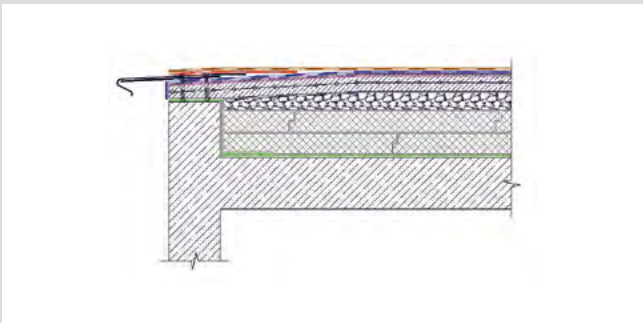
Устройство системы
